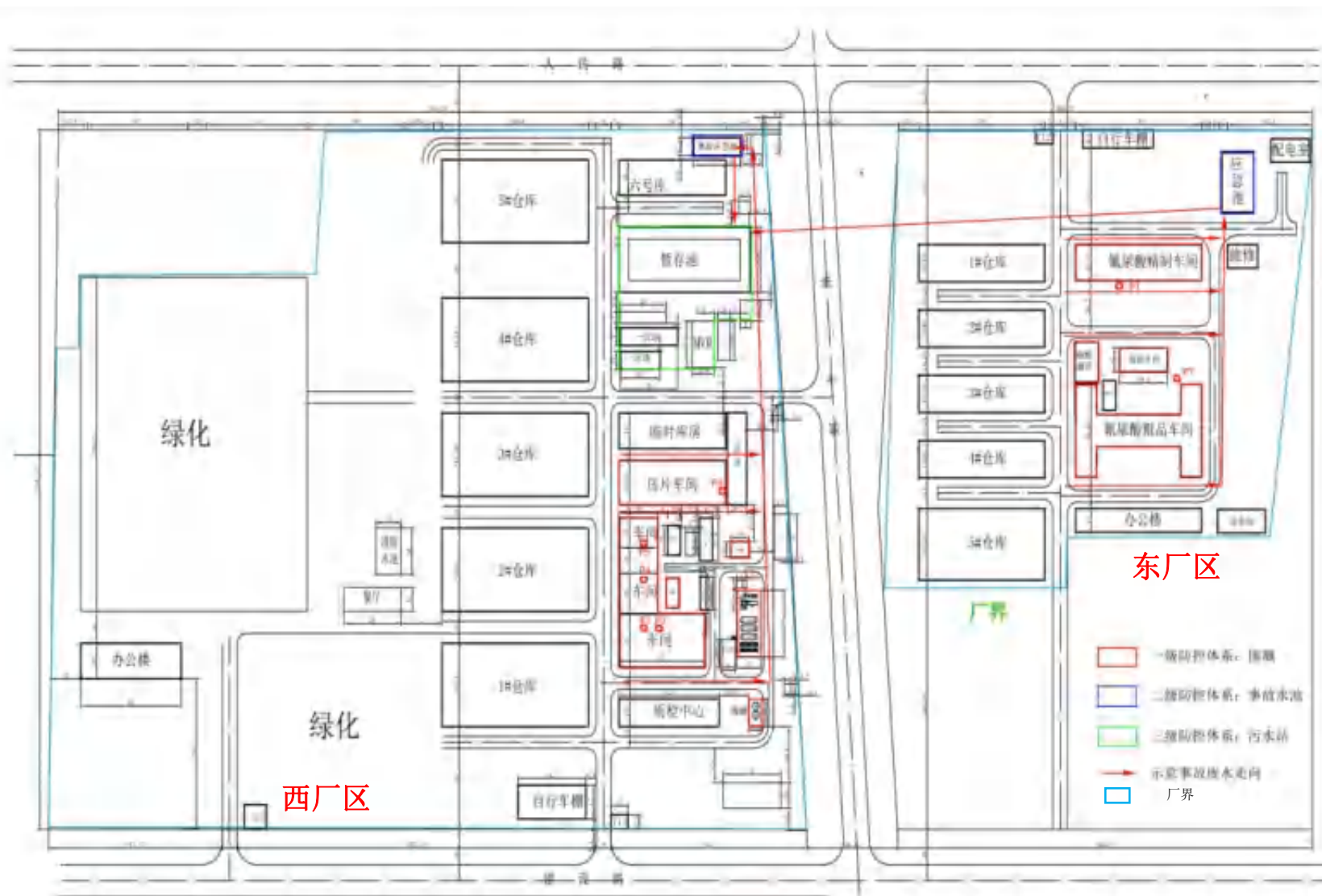
图2.2-1全厂总平面布置
