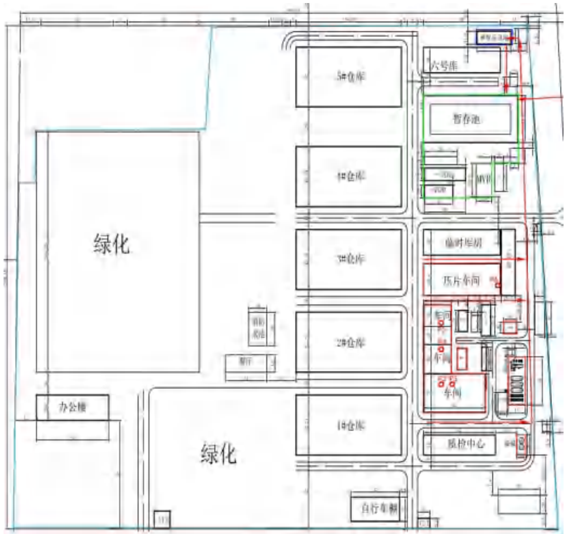
图2.2-3 平面布置图局部区域-西厂区
